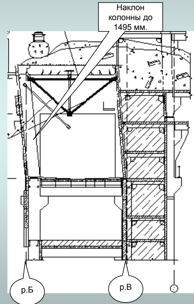
Разрез. Деаэрационная этажерка
